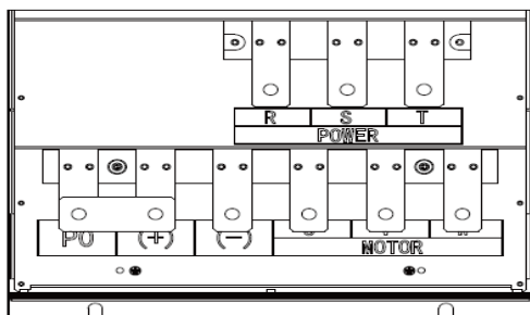
(h) 主回路功率端子 (200-220kW) 壁挂式
