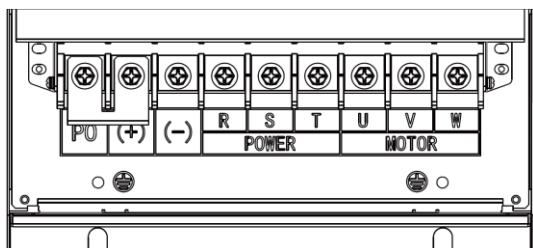
(e) 主回路功率端子 (55-75kW)
