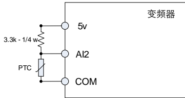
图 6.24 PTC 接线示例
