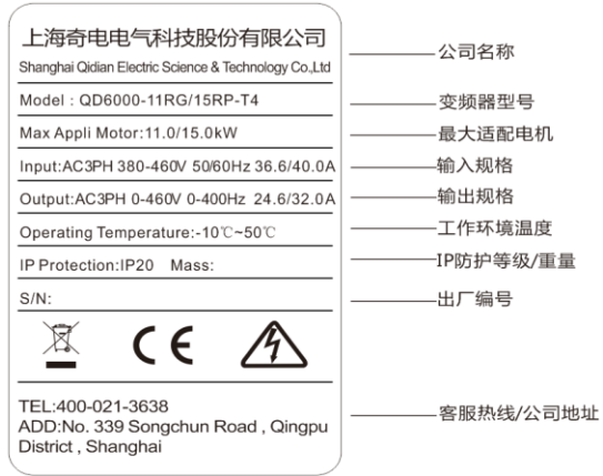
图 3.2 铭牌示例
