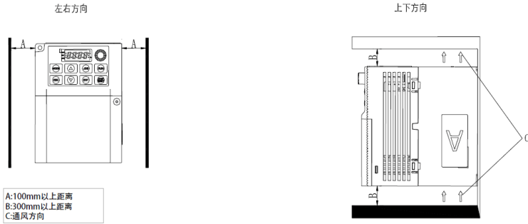
图 4.2 单台安装间距要求
