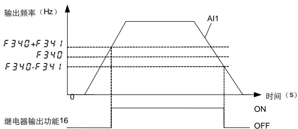
图 6.15 继电器输出-AI1 输入检出示意图
