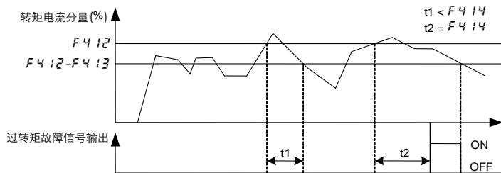
b) 过转矩故障输出信号示意图
