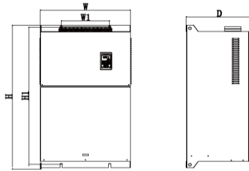
图 3.5 外形及安装尺寸示意图 (三相 355KW-500KW)
