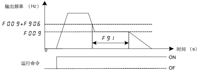
图 5.40 休眠模式进入
