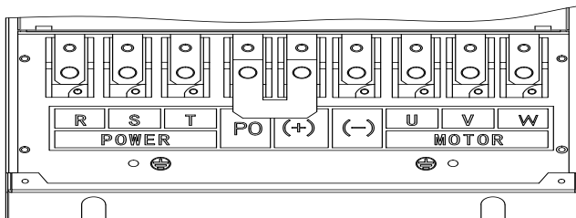
(d) 主回路功率端子 (45kW)
