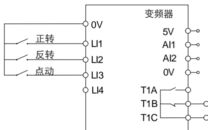
图 5.12 点动控制接线示意图
