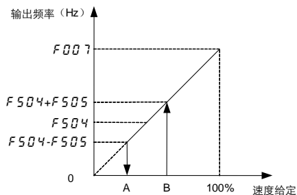
图 6.26 运行起始频率
