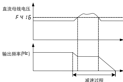
图 6.23 过压故障工作电平示意
