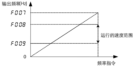
图 6.2 F007 , F008 , F009 和运行速度关系
