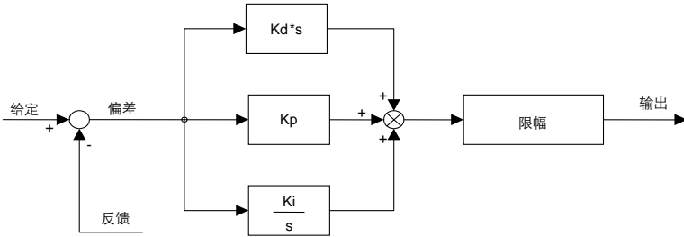
图 6.37 PID 调节器框图
