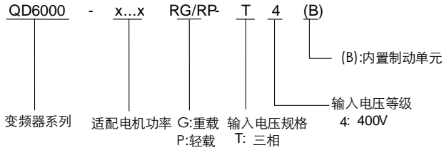
图 3.1 变频器型号说明示意图
