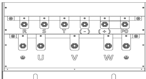
(j) 主回路功率端子 (355-500kW) 壁挂式
