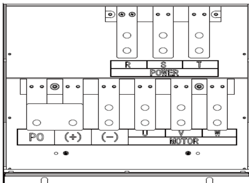
(i) 主回路功率端子 (250-315kW)
