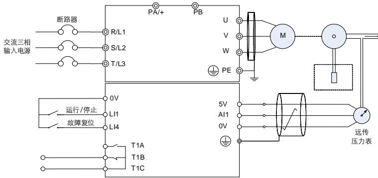
图 6.38 PID 外部连接示例
