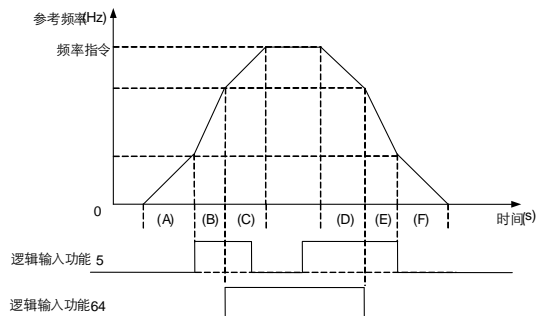
图 6.32 通过逻辑输入切换加减速曲线
