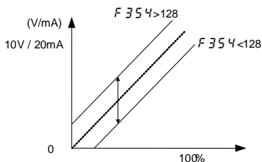
图 6.20 模拟输出曲线与 F354 关系
