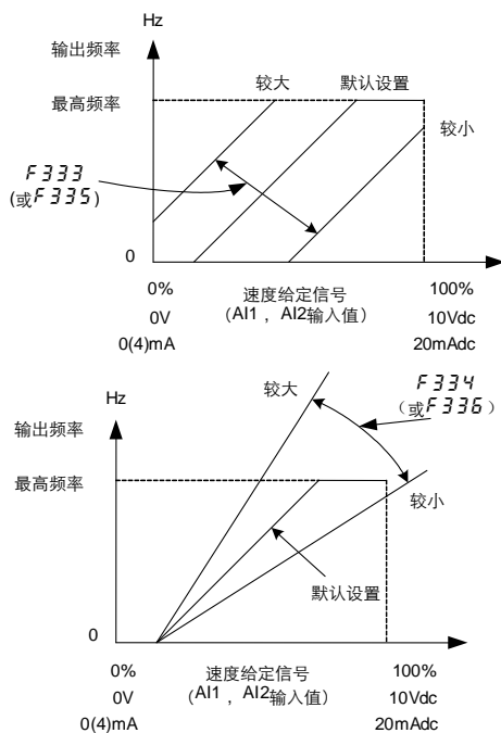
图 6.12 模拟输入校准
