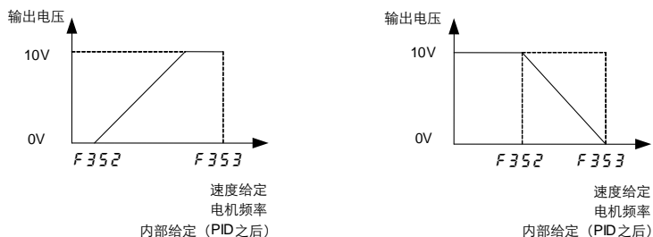
图 6.19 F352 和 F353 设置示意图
