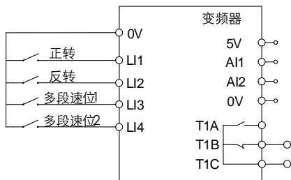
图 5.11 多段速控制接线示意图
