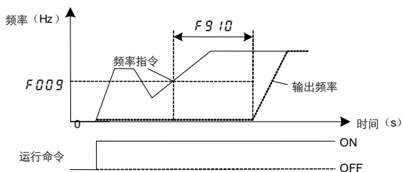
图 6.39 休眠唤醒示意图
