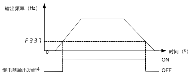
图 6.13 继电器输出-低速频率检出示意图
