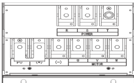
(g) 主回路功率端子 (132-185kW)
