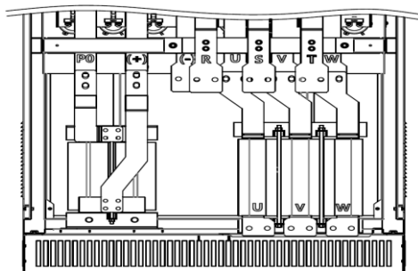
(k) 主回路功率端子 (560-800kW) 壁挂式
