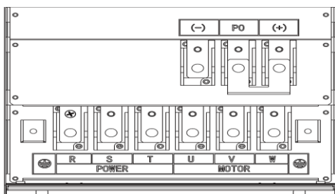
(f) 主回路功率端子 (90-110kW)
