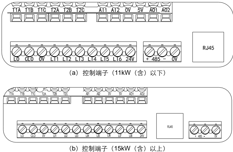
图 4.8 控制端子结构示意图
