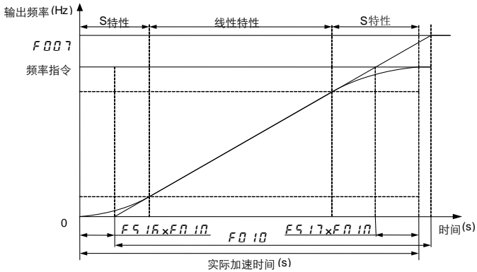
图 6.28 S 型曲线 1
