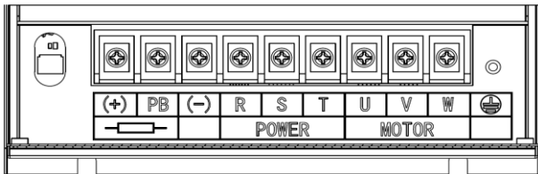
(c) 主回路功率端子 (30-37kW)
