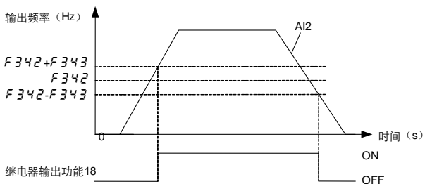
图 6.16 继电器输出-AI2 输入检出示意图
