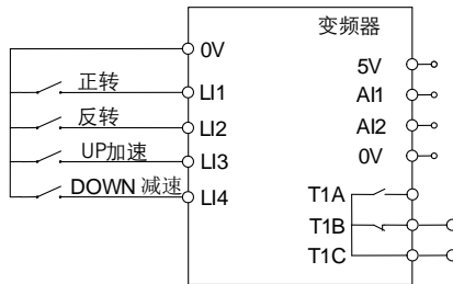
图 5.10 UP/DOWN 加减速接线示意图
