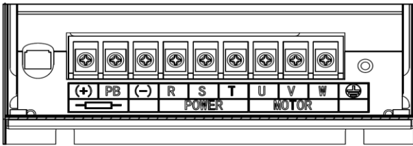
(b) 主回路功率端子 (15-22kW)
