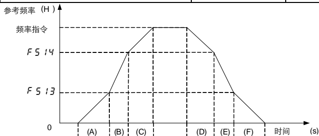
图 6.30 加减速曲线的自动切换
