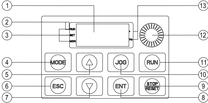
图 5.1 操作面板外形
