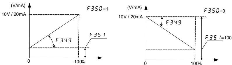
图 6.18 参数 F349 , F350 和 F351 设置示意图
