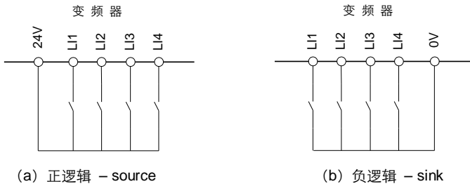
图 4.9 逻辑输入端子接线图
