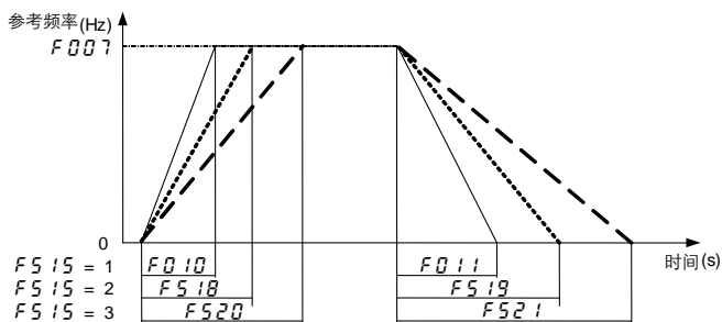
图 6.31 加/减速时间参数
