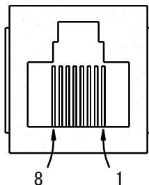
图 A.1 RJ45 正视图
