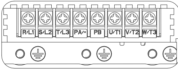
(a) 主回路功率端子 (11kW (含) 以下)
