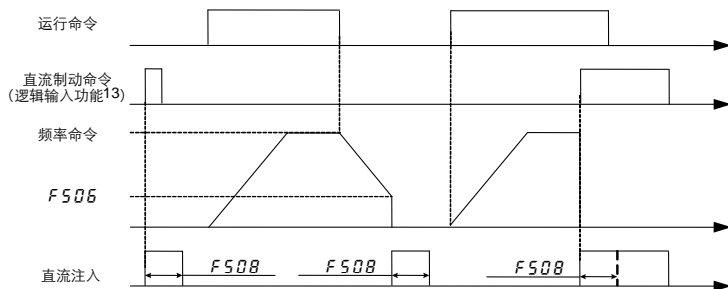
图 6.27 直流制动时序
