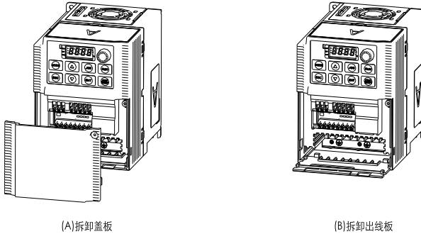
图 4.4 盖板、出线板的拆卸示意图
